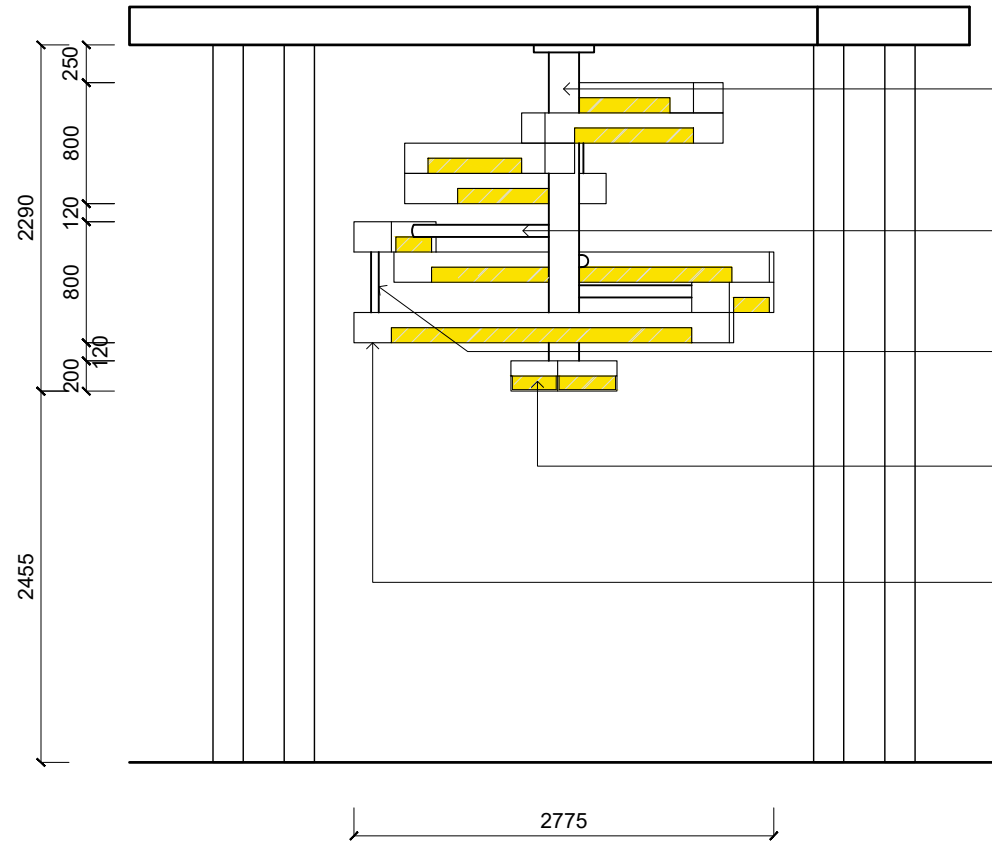
ELEVATION(EL-1) 1:50 PENDANT
