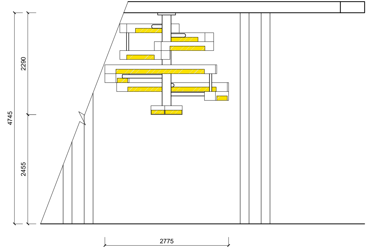
ELEVATION(EL-3) 1:50 PENDANT
