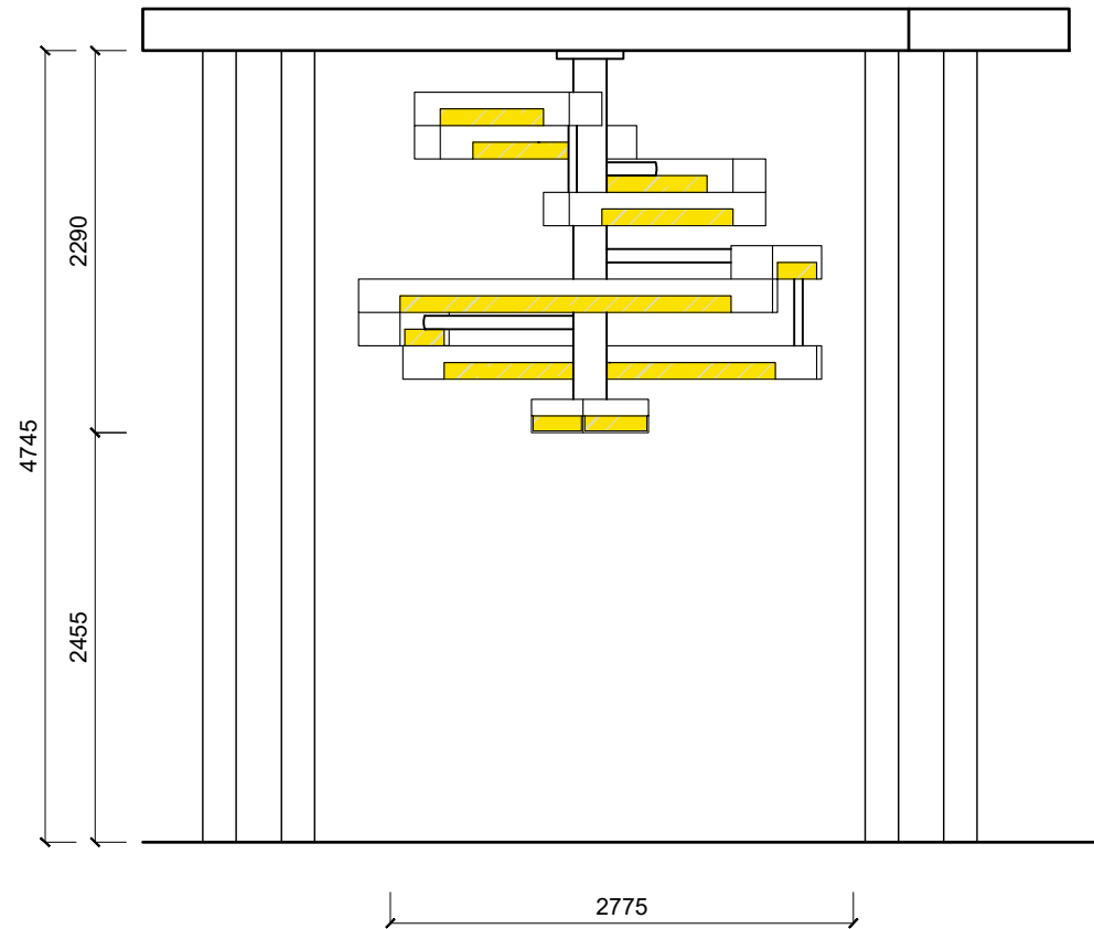
ELEVATION(EL-2) 1:50 PENDANT
