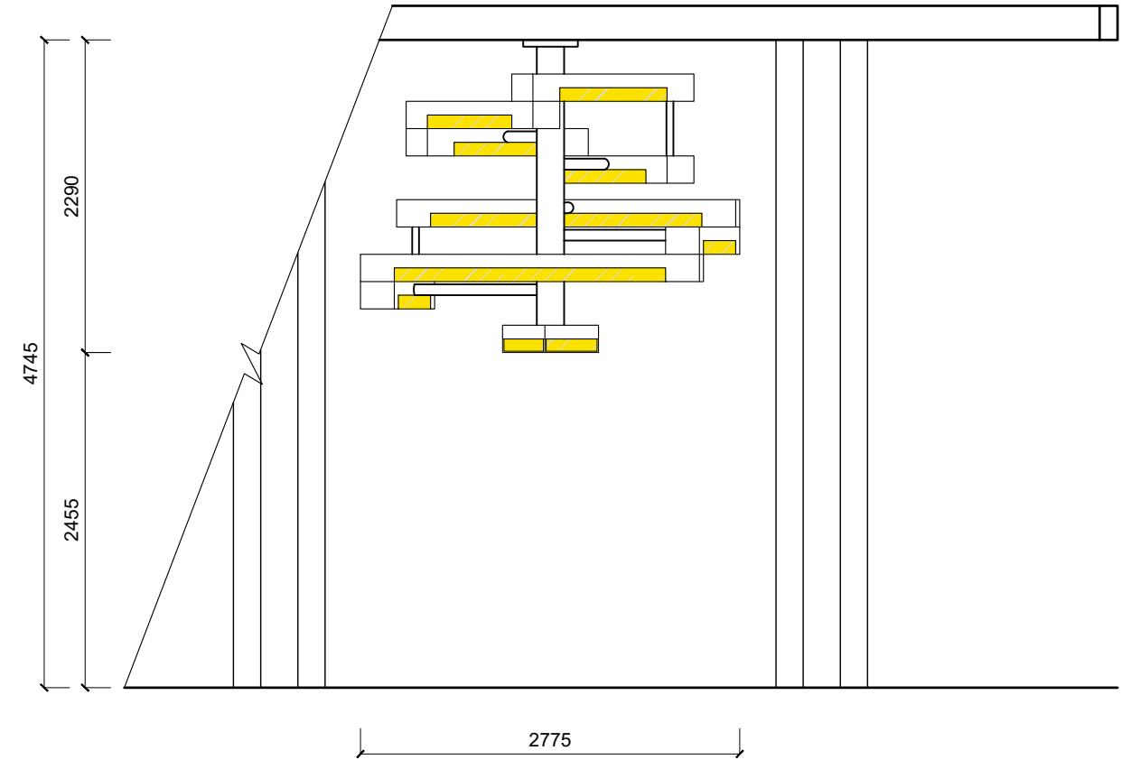
ELEVATION(EL-4) 1:50 PENDANT
