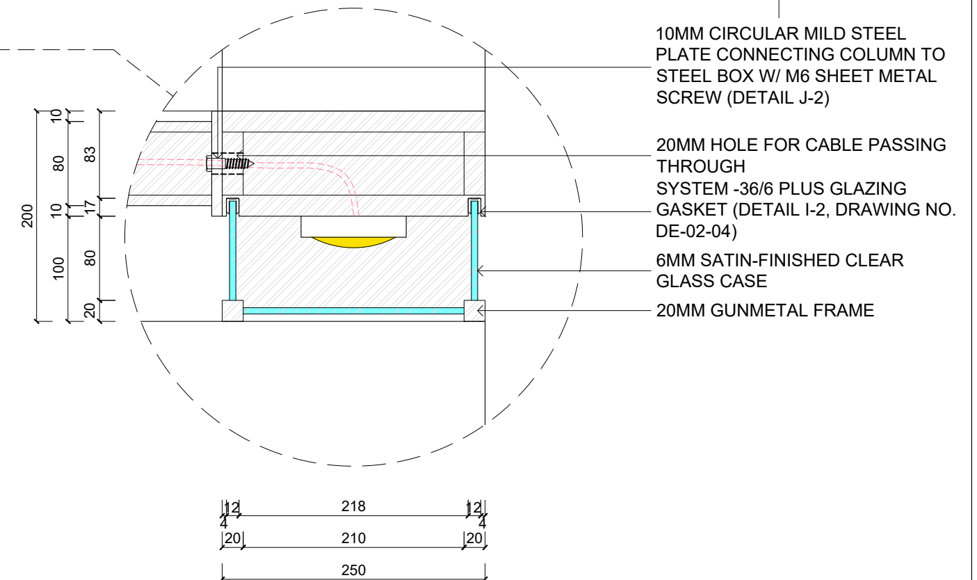
DETAIL J-1 1:5 PENDANT LIGHT BOX
